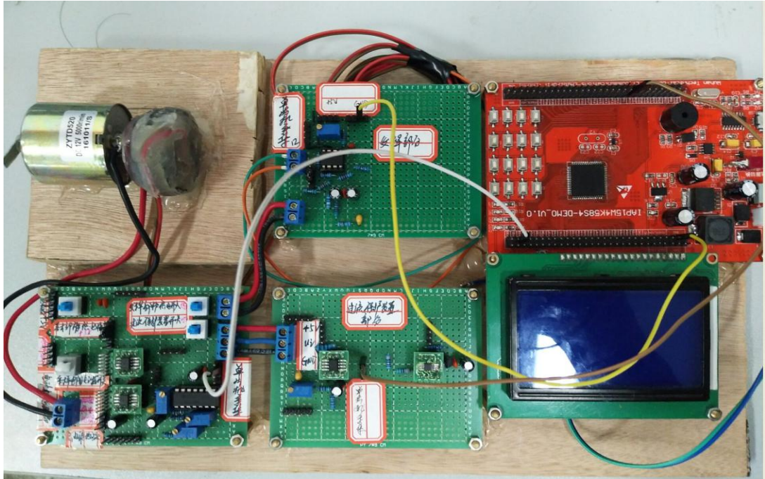
2017 年 8 月全国大学生电子大赛一直流电动机测速装置(全国一等奖)
